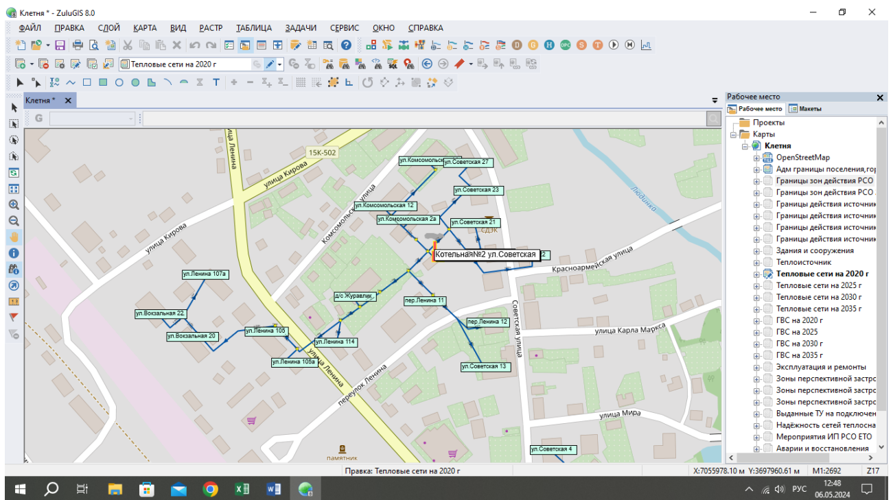
Рисунок 3.1. Электронная модель котельная пгт. Клетня, котельная №2, ул. Советская.
